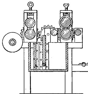
Parceling-Machine.
